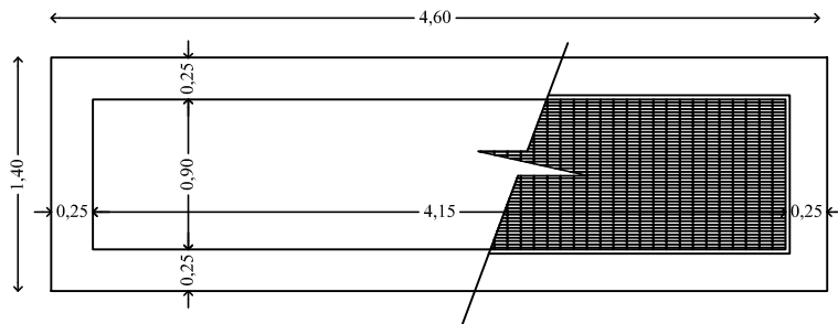
Pianta copertura pozzetto-canale
